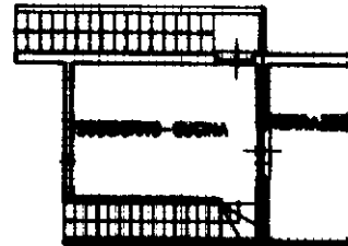
PIANTA PIANO PRIMO H.=2.70
